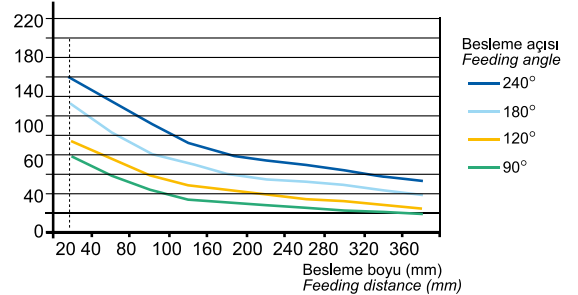
Sürekli çalıřma diagramı / Non-stop cycle diagram
